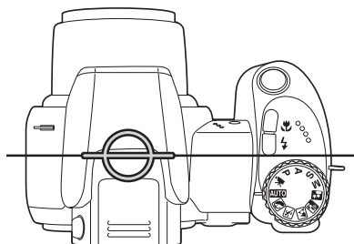
Posizione approssimativa del piano CCD
